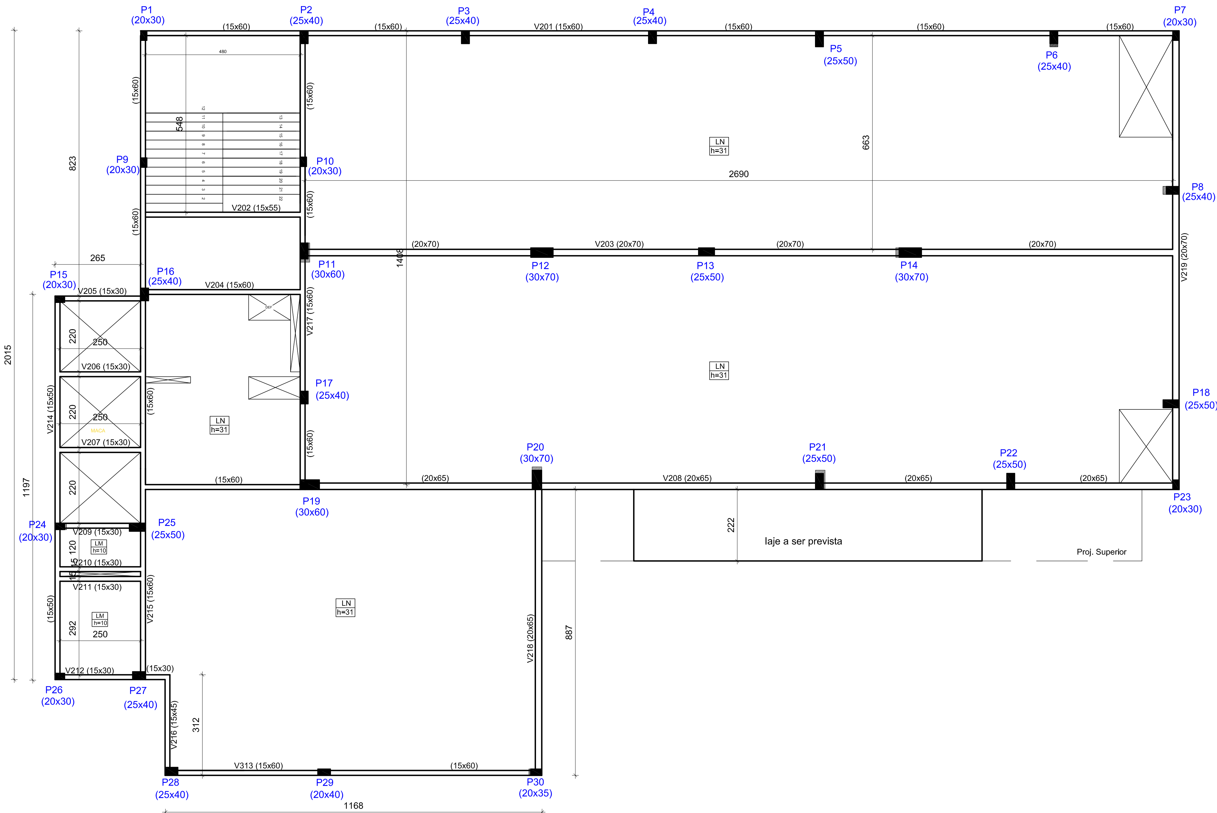
Planta de Fôrmas - 3º Pavimento Escala 1:50
